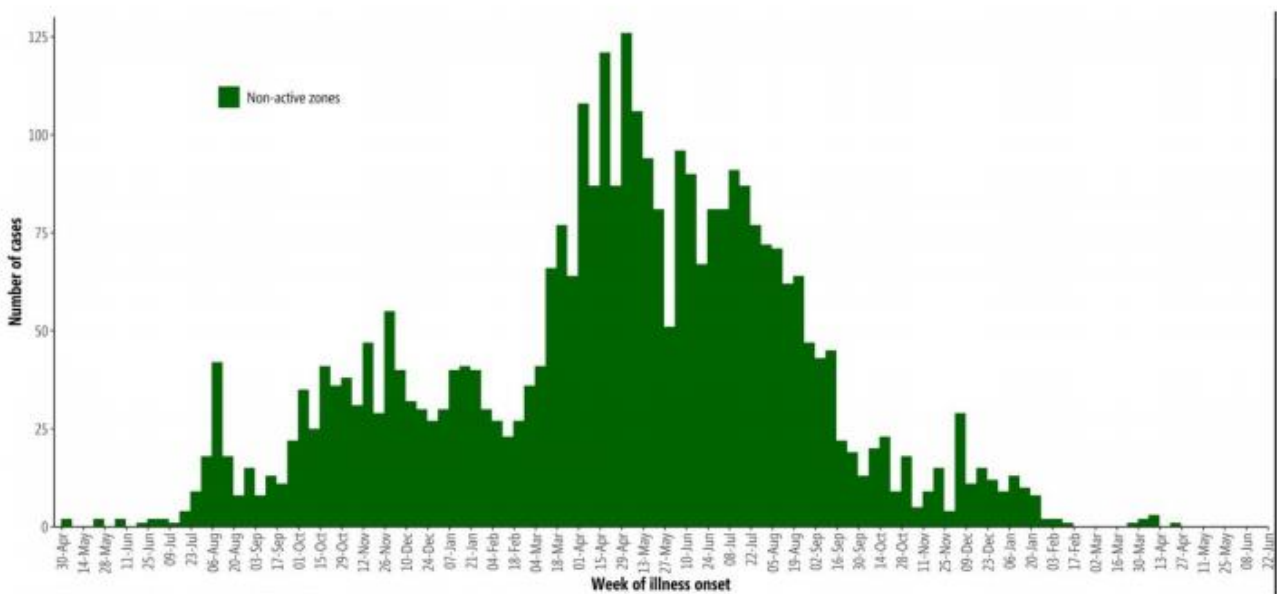
ภาพที่ 1 รายงานสัปดาห์ตามวันที่เริ่มป่วย ในเขตสุขภาพ ของสาธารณรัฐประชาธิปไตยคองโก ณ วันที่ 21 มิถุนายน 2563
