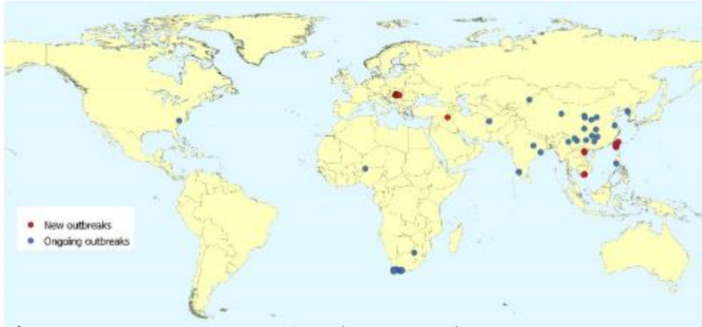
ภาพที่ 1 การระบาดของสัตว์ปีกใหม่ อย่างต่อเนื่อง ระหว่างวันที่ 29 พฤษภาคม – 18 มิถุนายน 2563
