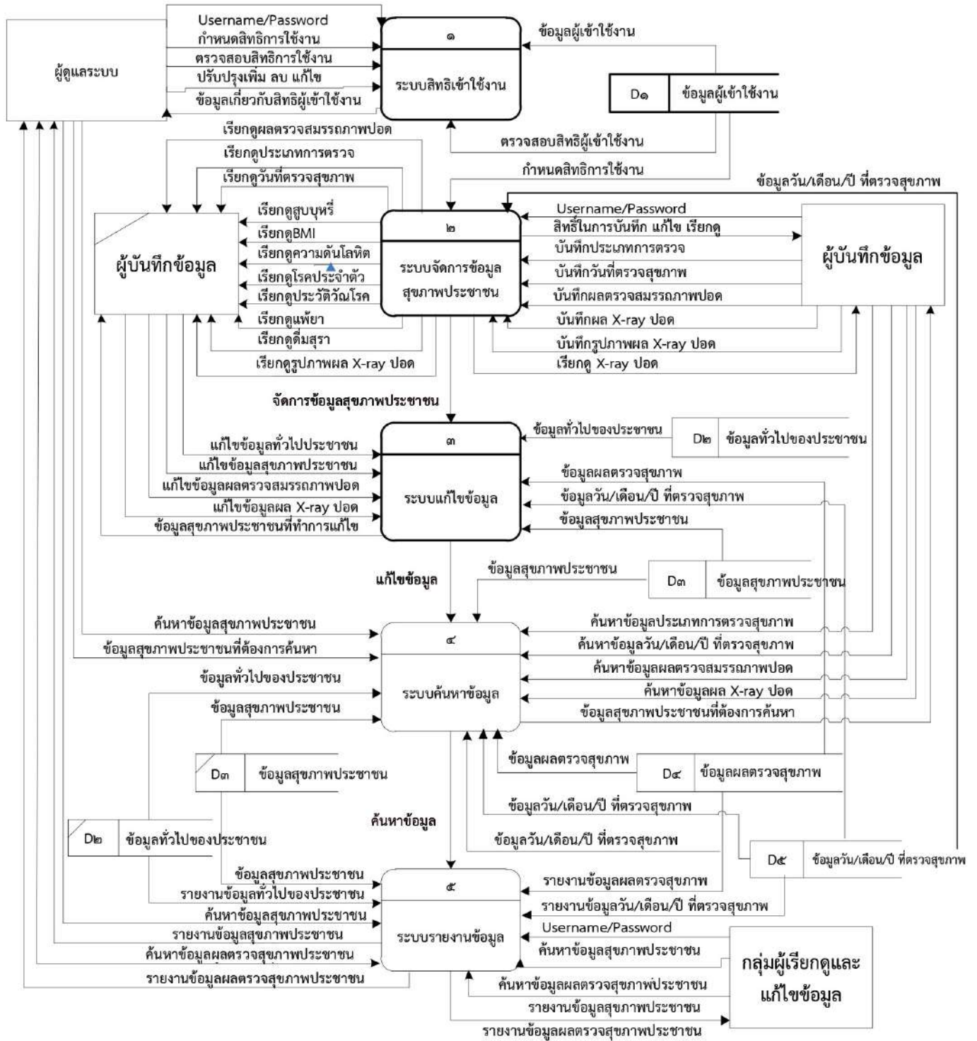
แผนการไหลของข้อมูล DFD: Data Flow Diagram Level ๑ โปรแกรม Naphralarn Health Program ๔.๐
